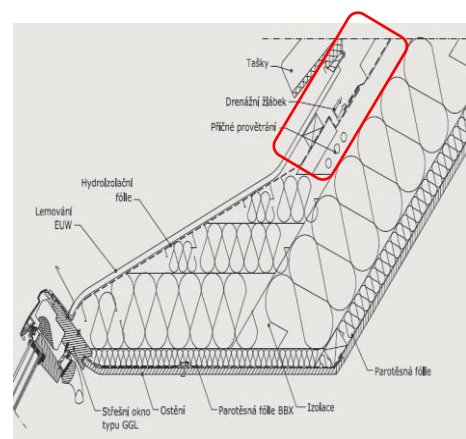
Obr. 2) průřez kontralatí, zdroj www.velux.cz
