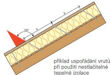
Obr. 3) schéma uspořádání šikmých vrutů Twin UD
