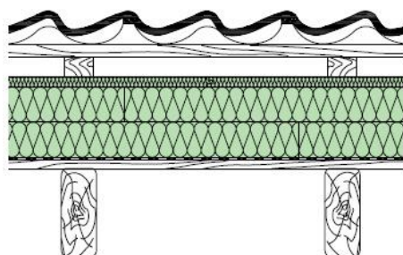
Obr. 7) Schéma a popis experimentálně ověřované konstrukce
