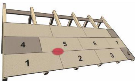
Obr 2) : Schéma kladení desek PAVATEX na krokve, spoje ve směru krokve „na vazbu“
