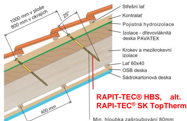
Obr. 4) : Schéma vruty RAPI-TEC®
