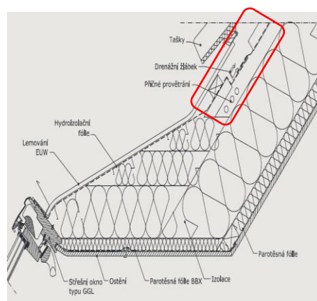
Obr. 3) přerušení kontralatí, zdroj www.velux.cz
