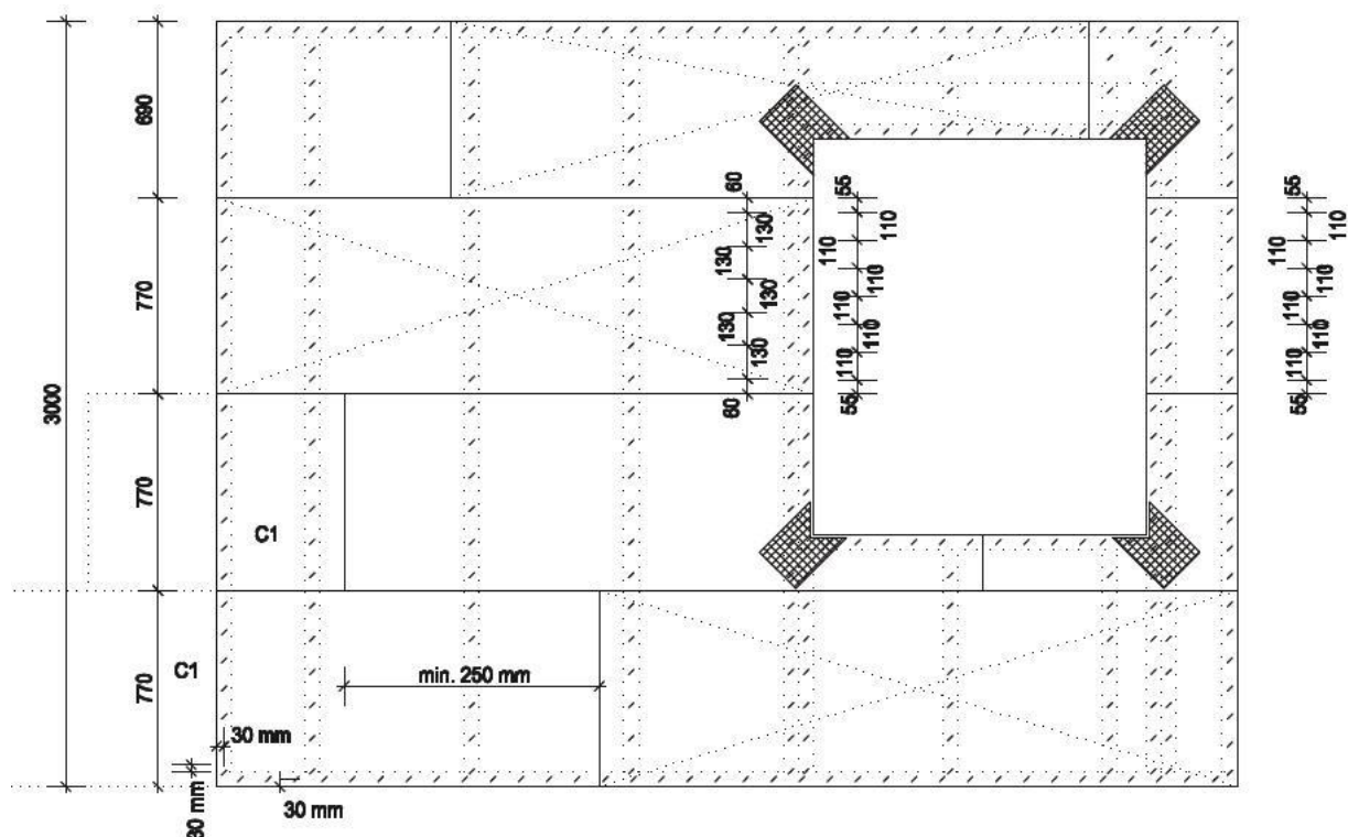
Obr. 7: Schéma kladení desek rozměru 770 mm na nosnou konstrukci včetně rozmístění spon
