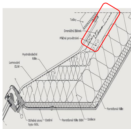
Obr. 5) přerušení kontratátí, zdroj www.velux.cz
