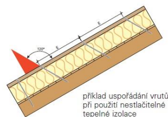
Obr. 7) : schéma uspořádání šikmých vrutů Twin UD
