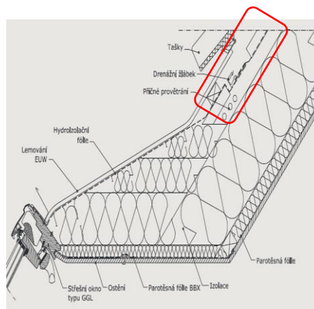
Obr. 5) přerušování kontratletí, zdroj www.velux.cz
