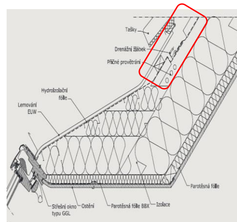
Obr. 2) přerušení kontralatě, zdroj www.velux.cz
