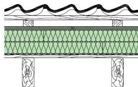
Obr. 7) Schéma a popis experimentálně ověřované konstrukce
