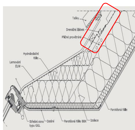
Obr. 2) přerušení kontralaty, zdroj www.velux.cz
